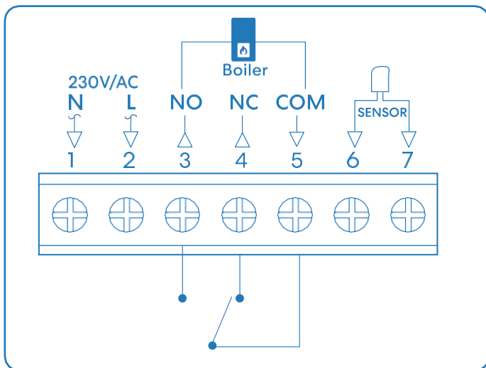
Vytápěcí systém s kotlem (ovládání kotle pomocí termostatu).
