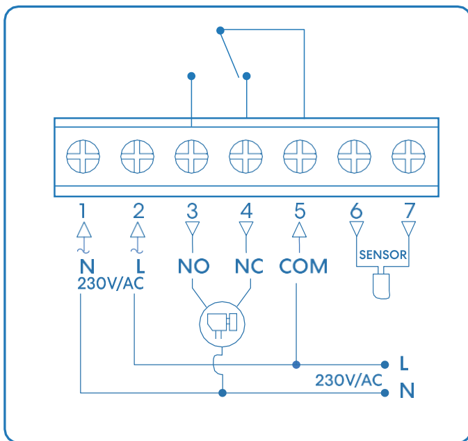
Systém vodního podlahového vytápění (ovládání tepelného pohonu pomocí termostatu, podporuje dvou vodičové i třívodičové pohony).
